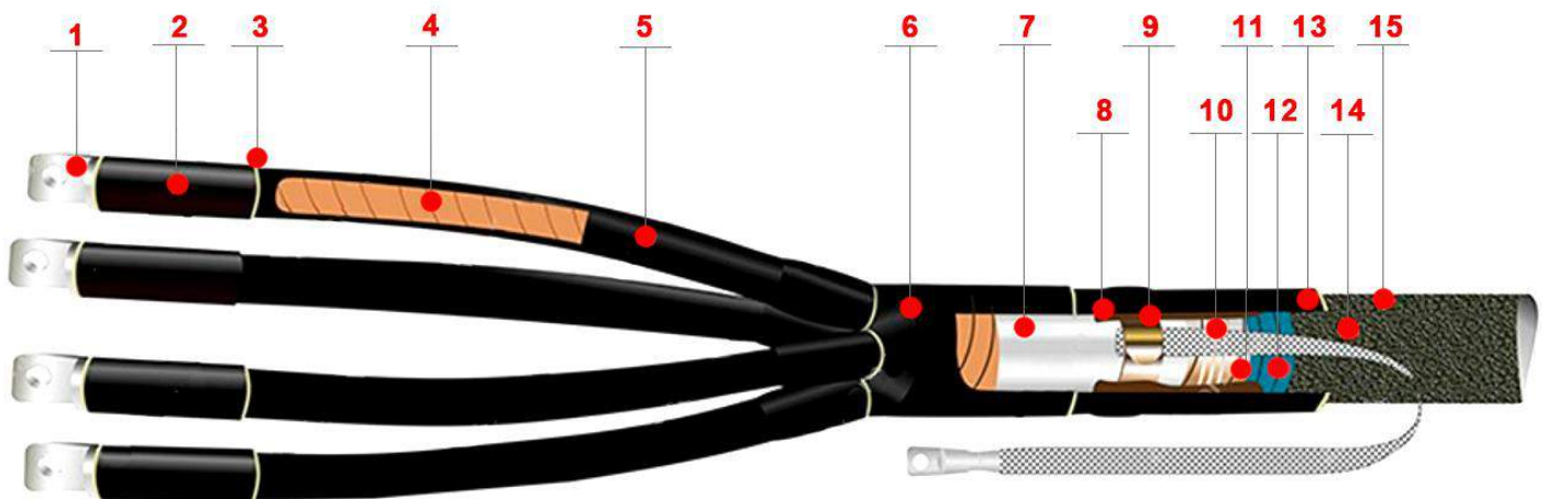
Муфта 4КВтп 1 стандартна комплектація
